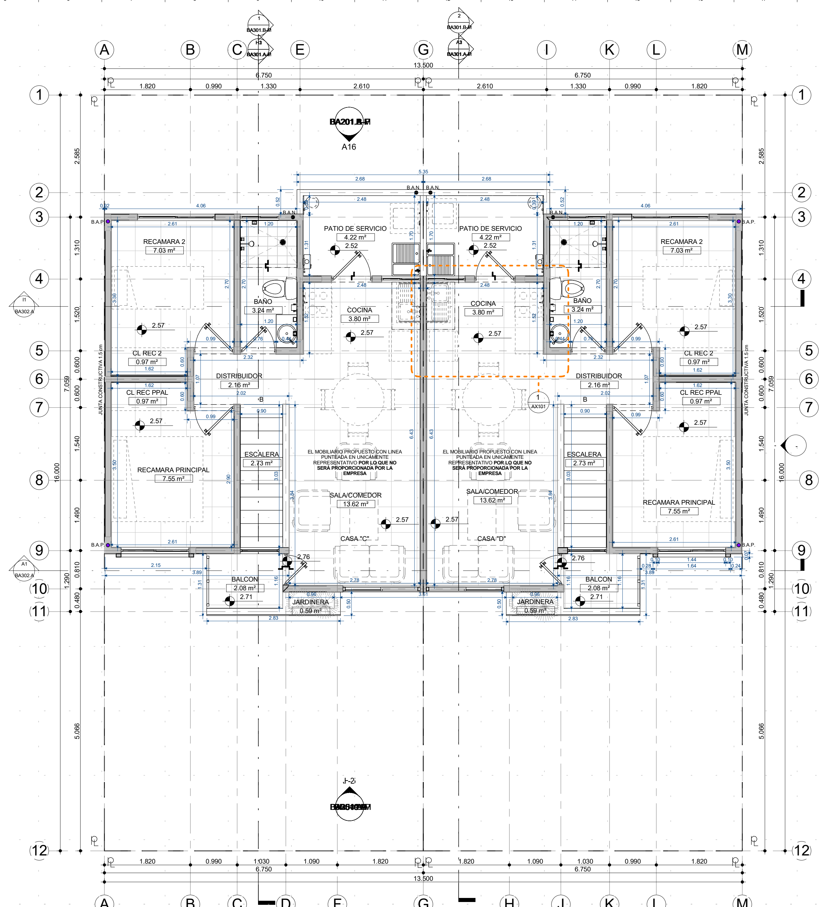
A1 ARQ_PLANTA ALTA OPCION "A" 1:50
